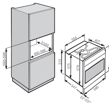
Esquema geral dos fornos
