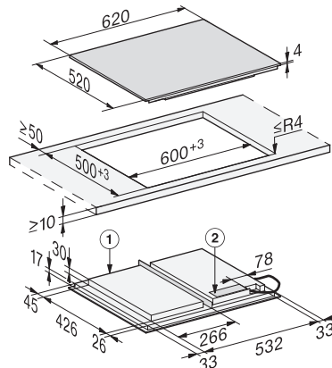
Instalação sobre a bancada (KM 7667 FL)
