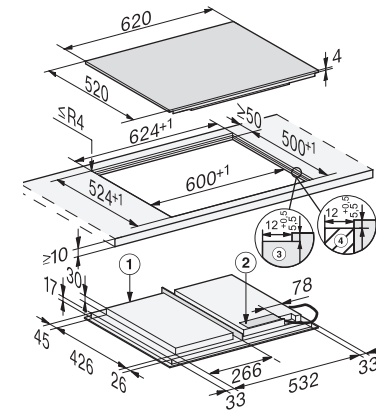
Instalação à face (KM 7667 FL)
